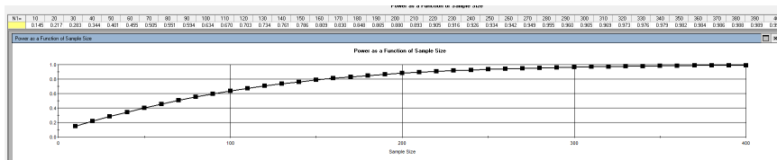
شکل ۱: نمودار برآورد حجم نمونه SPSS SAMPLE POWER
